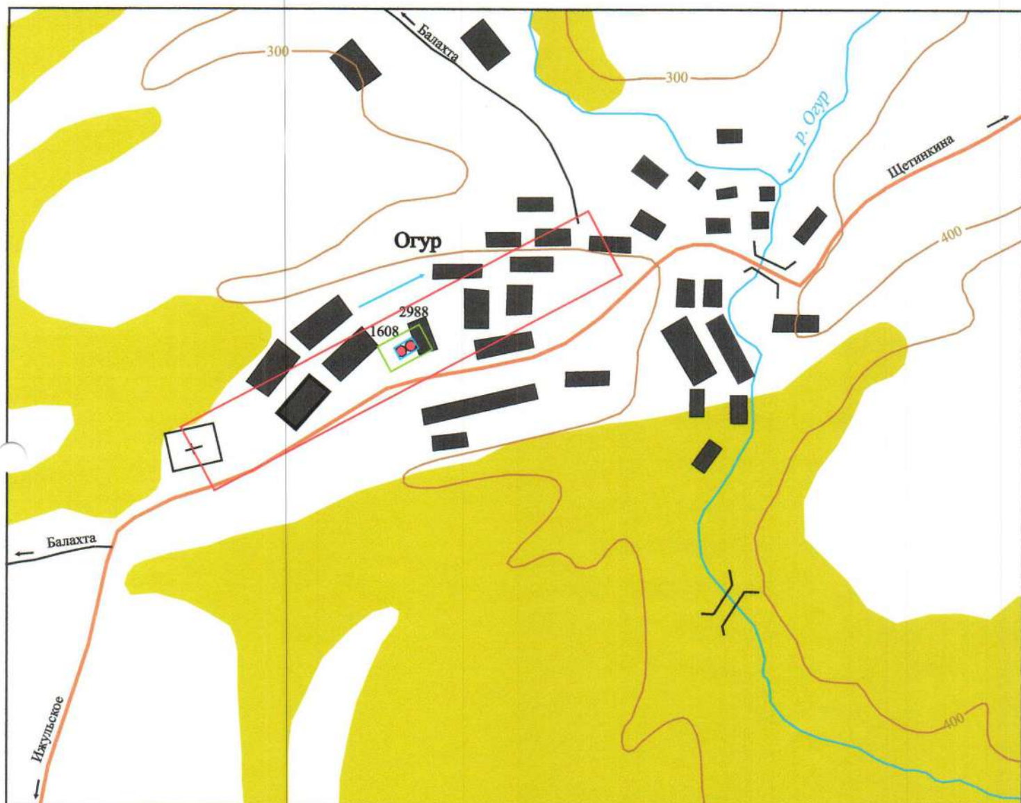
Рис. 3 Схема расположения зоны санитарной охраны водозаборных скважины 1608 и 2988
