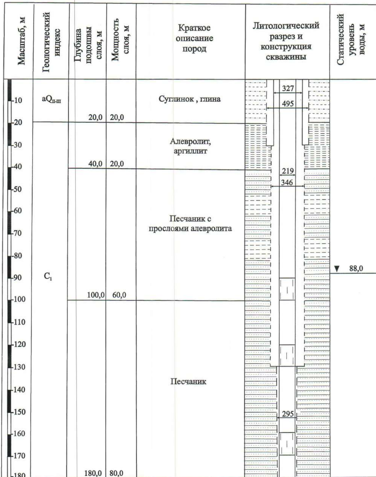
Рис. 2 Геолого - технический разрез водозаборной скважин 2988
