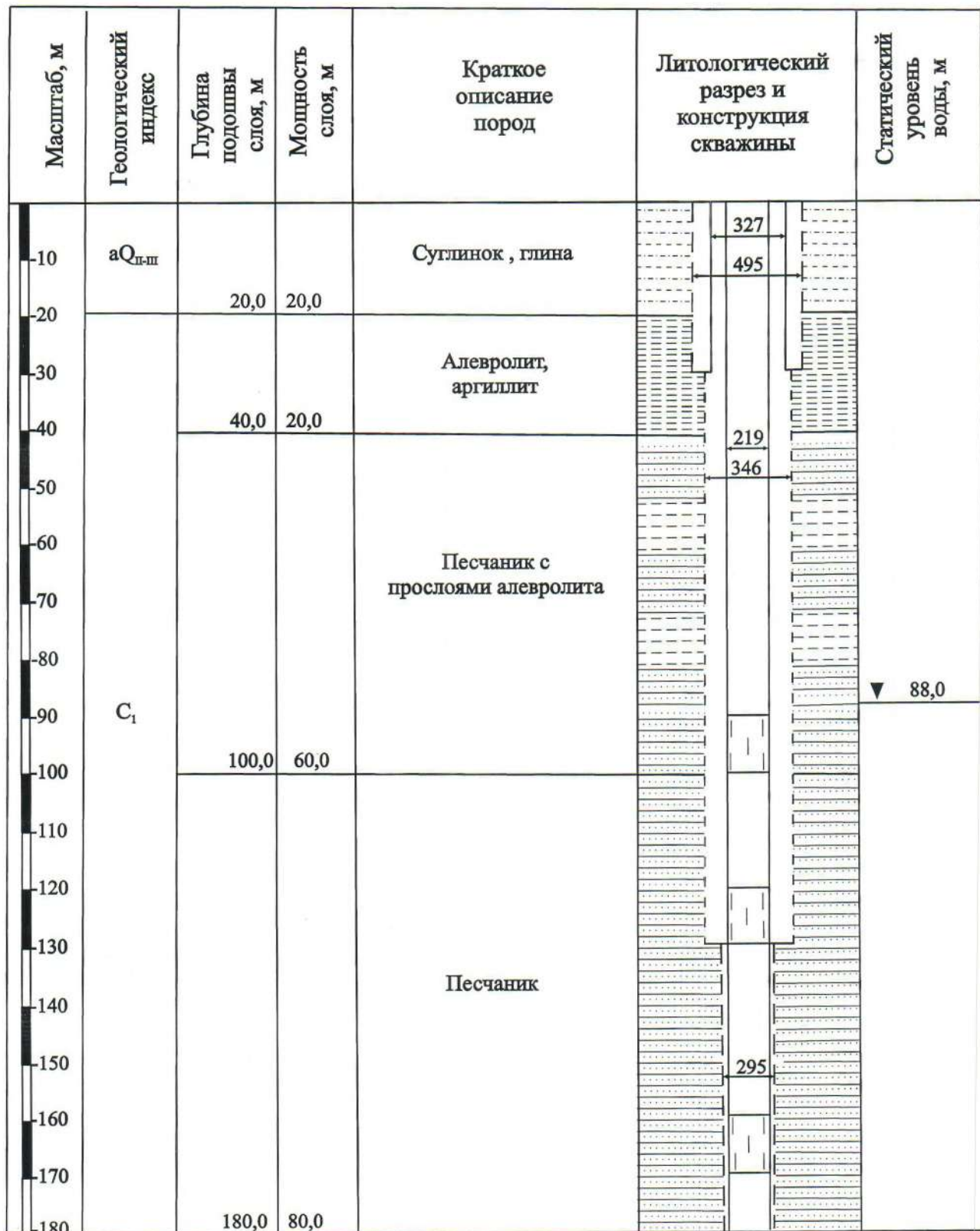
Рис. 2 Геолого - технический разрез водозаборной скважин 1608
