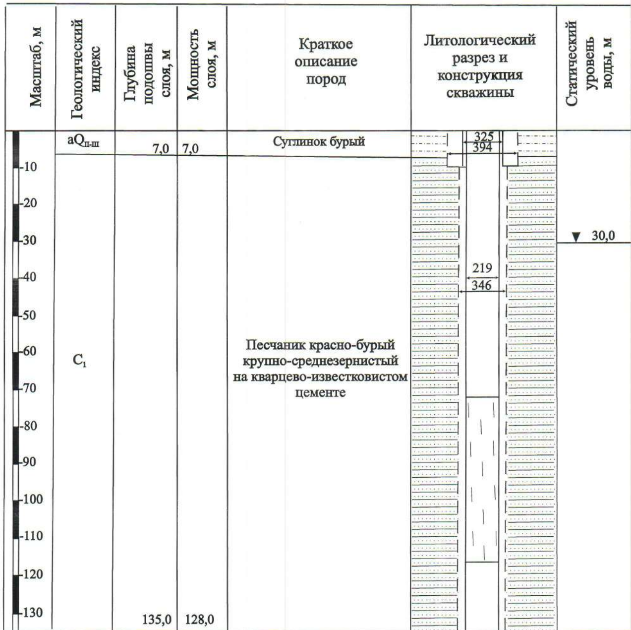
Рис. 2 Геолого - технический разрез водозаборной скважины 587
